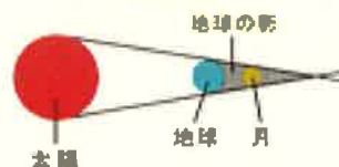
月食のしくみ
